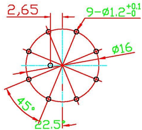
线路板开孔尺寸
