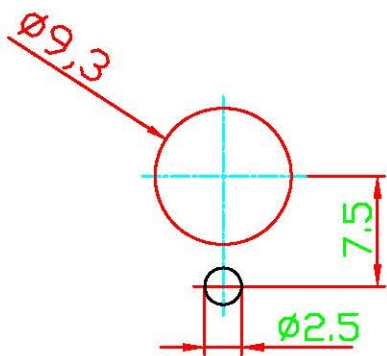
面板开孔尺寸
