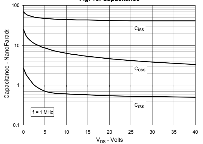
Fig. 10. Capacitance
