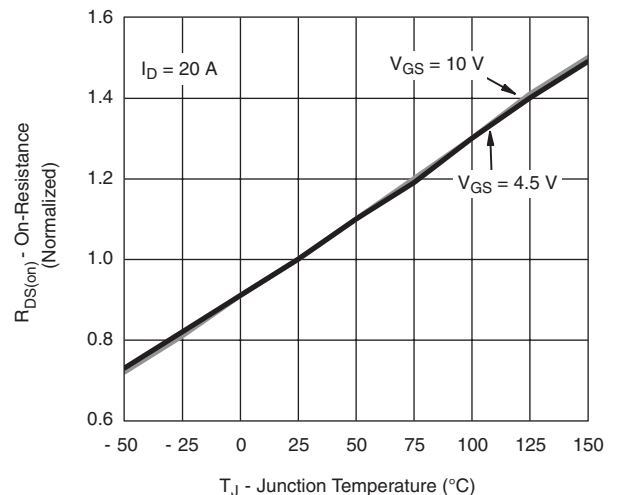
I_D = 20\text{ A} V_{GS} = 10\text{ V} V_{GS} = 4.5\text{ V}
